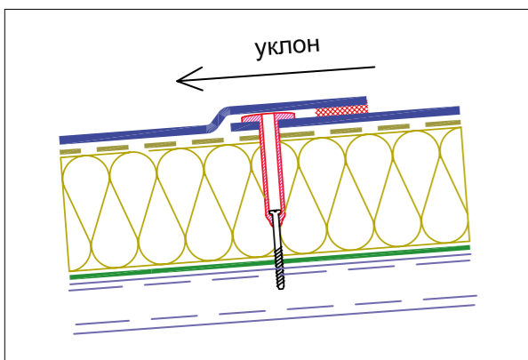
Рис. 3.4.4. Встречный шов
