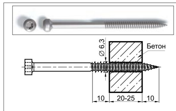
Рис. 2.10.1 Саморез по бетону \varnothing 6,3 мм
