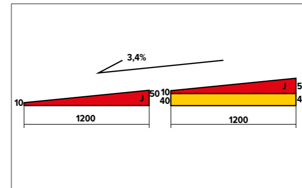
Рис. 3.3.14 Схема укладки контруклона LOGICPIR SLOPE 3,4 %
