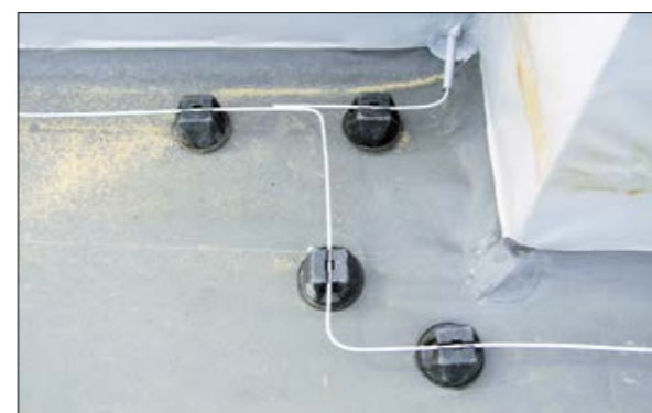
Рис. 4.8.13 Молниезащита ТЕХНОНИКОЛЬ
