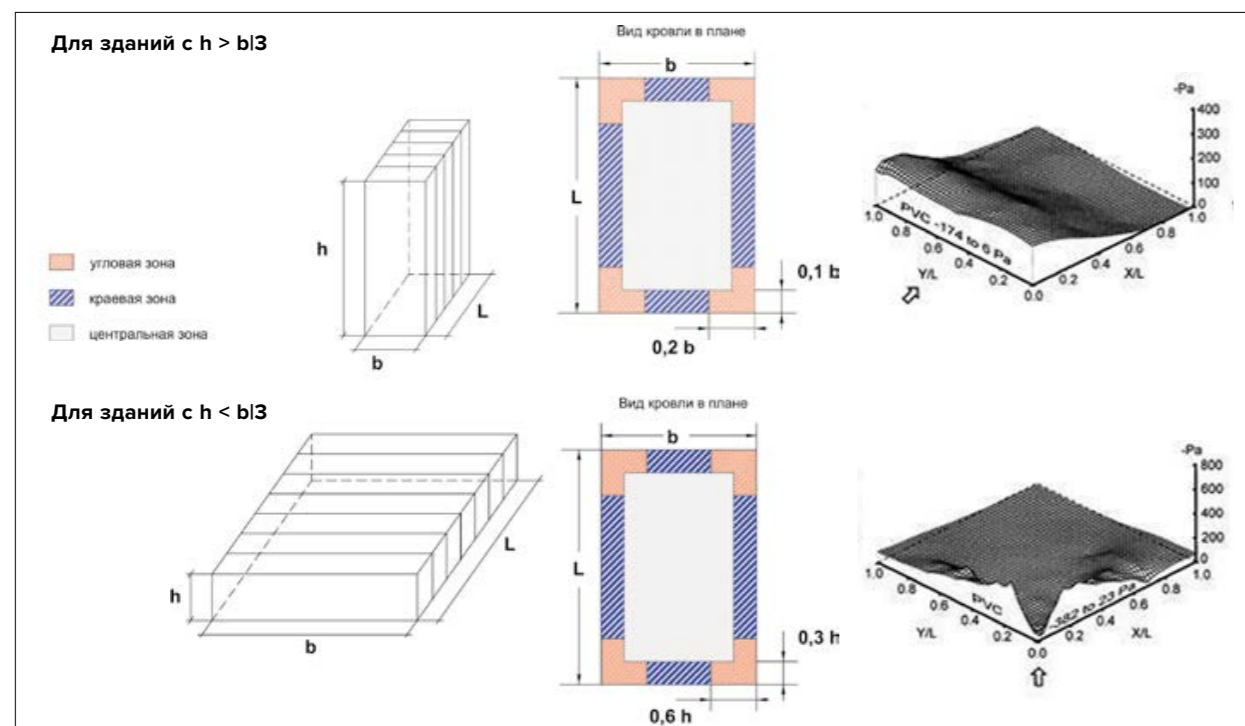
Рис. 3.5.1 Деление кровли на зоны ветровой нагрузки
