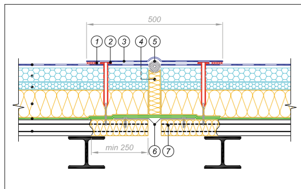
Рис. 3.6.2 Упрощенная конструкция деформационного шва
