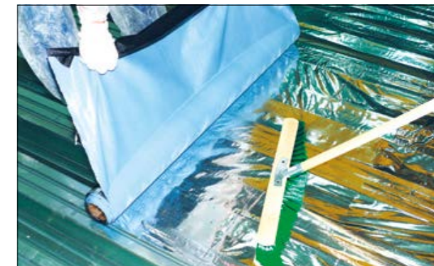
Рис. 3.1.10 Пароизоляция Паробарьер С укладывается вдоль верхних полок профнастила, снимается защитная пленка и материал приклеивается к основанию
