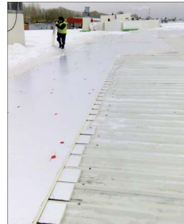
Рис. 2.11.1 Ремонт кровельной сэндвич-панели
