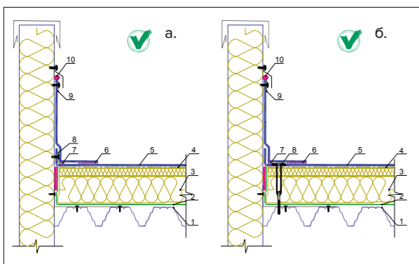
Рис. 3.6.6 Устройство классического примыкания кровельного ковра к вертикальной поверхности
