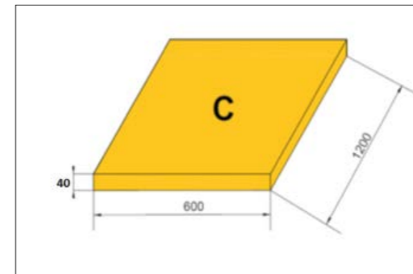
Рис. 3.3.13 Геометрия плит для создания контруклона LOGICPIR SLOPE 3,4 %
