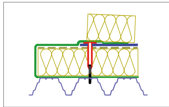
Рис. 3.1.8 Временная защита теплоизоляции от намокания
