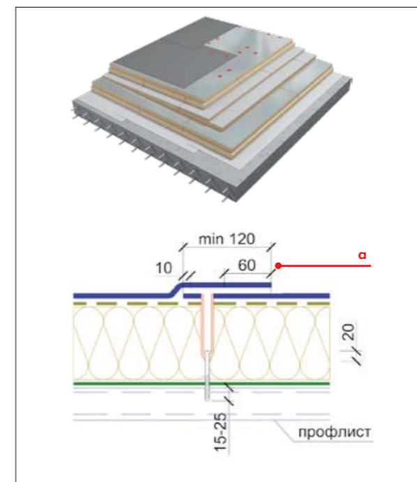
Рис. 3.5.6 Механическое крепление кровельного ковра
