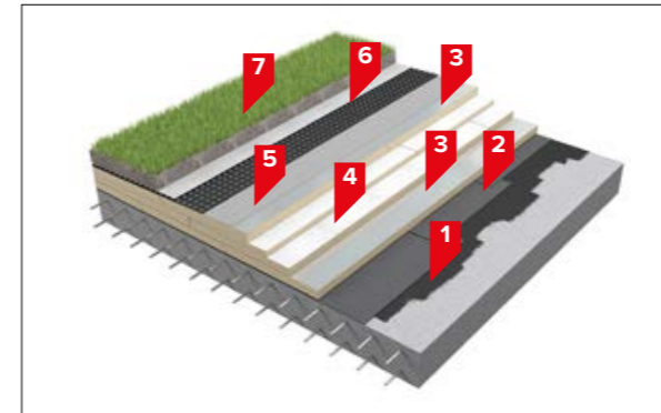
Рис. 2.7.6 Система полимерной «зеленой» кровли
