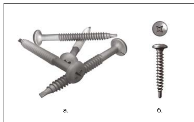
Рис. 3.5.11 Кровельный саморез сверлоконечный ТЕХНОНИКОЛЬ. а. Ø 4,8; б. Ø 5,5
