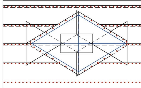
Рис. 3.3.11 Укладка ПВХ-мембраны в разуклонке из клиновидных плит
