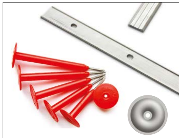
Рис. 3.5.9 Распределители нагрузки для механического крепления. Пластиковые тарельчатые телескопические элементы (слева), металлические тарельчатые прижимные держатели (справа внизу), линейные прижимные держатели (справа сверху)
