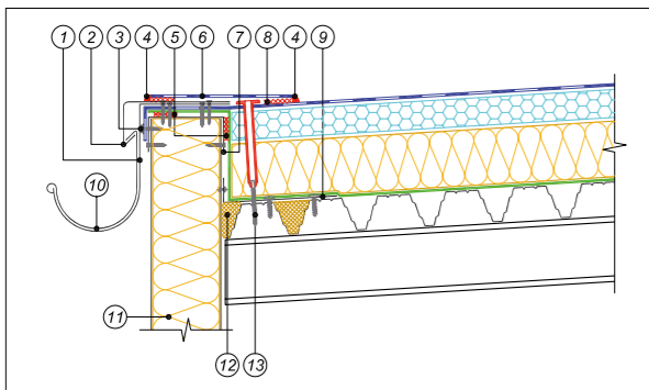
Рис. 4.8.3 Решение карнизного свеса с использованием ламинированного металла
