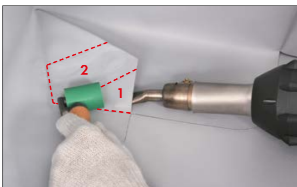
15. Приварите последовательно сегменты «конверта» 1 и 2.
