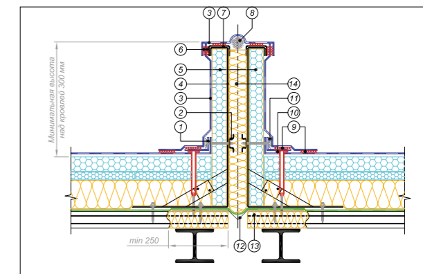
Рис. 3.6.1 Конструкция деформационного шва
