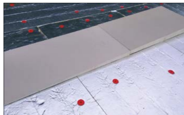
Рис. 3.3.12 Изображение LOGICPIR SLOPE с уклоном 1,7 %
