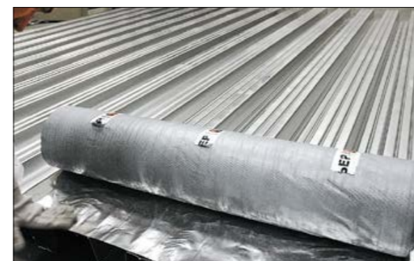
Рис. 3.1.11 Укладка пароизоляционного материала по профлисту
