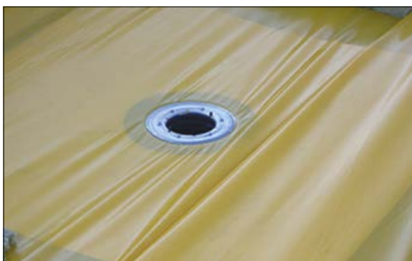
Рис. 3.6.10 Последовательность установки двухуровневой воронки
