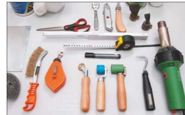
Рис. 5.1.1 Комплект оборудования для производства работ по укладке мембран
