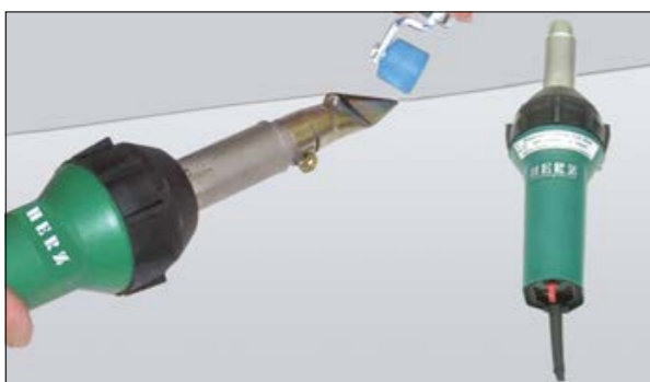
Рис. 4.8.11 Ручное сварочное оборудование
