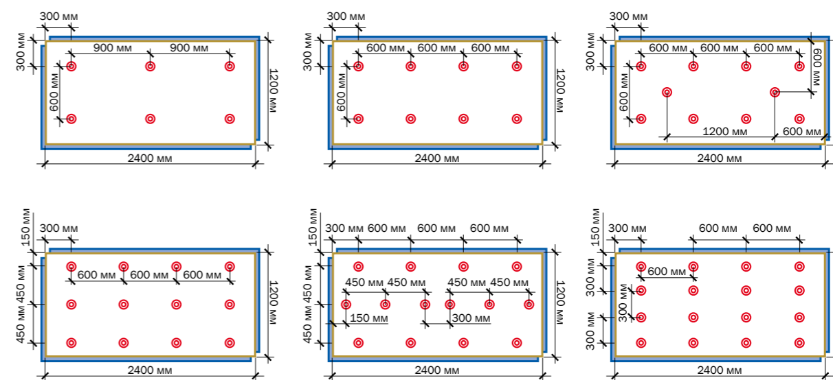
Рис. 2.3.5 Схемы крепления плит LOGICPIR при индукционной системе крепления
