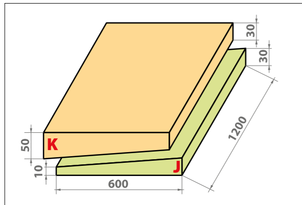
Рис. 3.3.9 Клиновидные уклонообразующие плиты К и J из XPS
