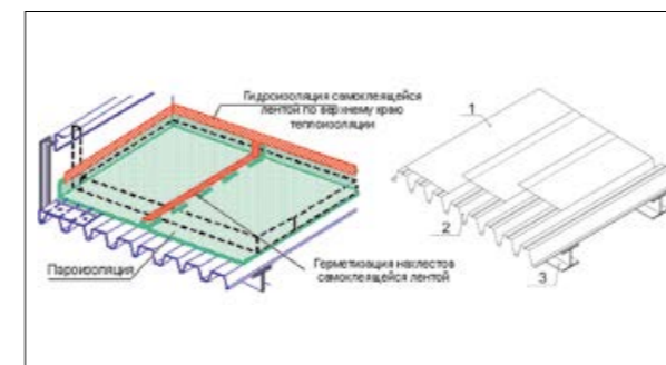
Рис. 3.1.3 Правильная склейка перехлестов пароизоляции в системе с основанием из профлиста
