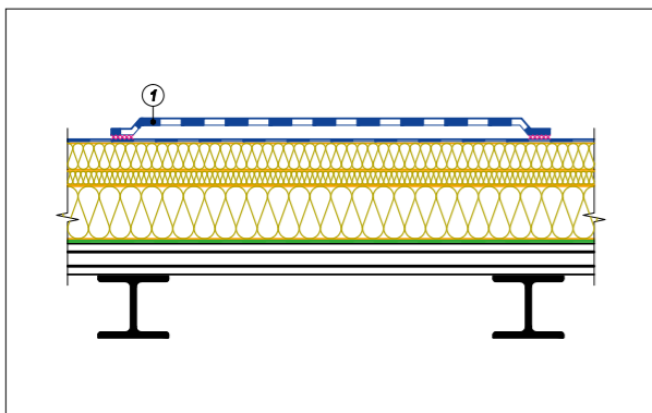
Рис. 3.6.6 Современный вариант устройства пешеходных дорожек из готовых элементов LOGICROOF WalkWay Puzzle
