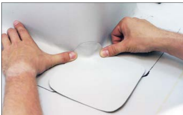
Рис. 3.4.1 Применение неармированной ПВХ мембраны при устройстве внешнего угла.
