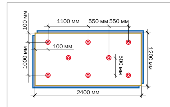
Рис. 2.2.4 Рекомендуемая схема крепления плит теплоизоляционных LOGICPIR PROF
