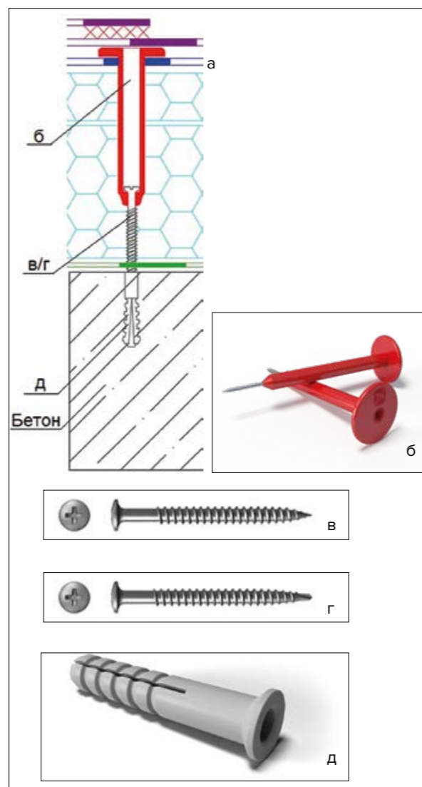
Рис. 2.10.2 Система механического крепления ТЕХНОНИКОЛЬ: а – общий вид смонтированного крепежа в бетонное основание, б – телескопический крепеж, в – саморез остроконечный \varnothing 4,8 мм, г – саморез сверлоконечный \varnothing 4,8 мм, д – анкерный элемент \varnothing 8 мм
