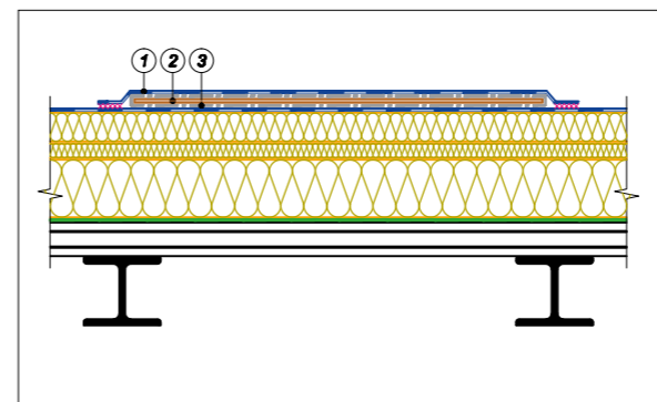
Рис. 3.6.5 Устройство пешеходных дорожек
