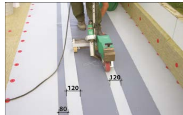
Рис. 3.6.9 Приварка автоматом полосы
