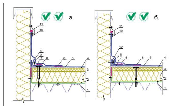
Рис. 3.6.7 Устройство примыкания кровельного ковра к вертикальной поверхности с усиленным креплением
