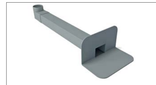
Рис. 4.7.5 ПВХ воронка парапетная 65x100мм длиной 550мм с отводом \varnothing 100 мм
