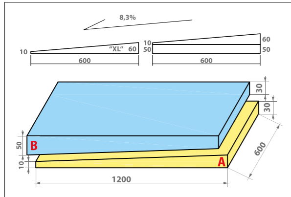
Рис. 3.3.8 Клиновидные уклонообразующие плиты А и В из XPS или PIR
