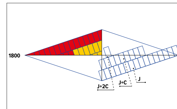
Рис. 3.3.15 Пример раскладки разуклонки плит LOGICPIR SLOPE 3,4 % для формирования уклона
