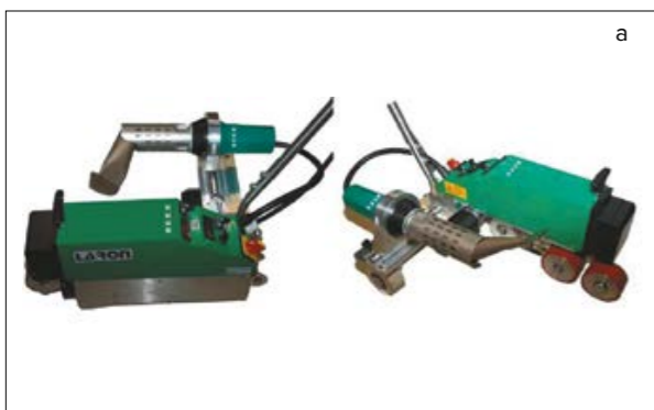
Рис. 4.8.12 Автоматическое сварочное оборудование
