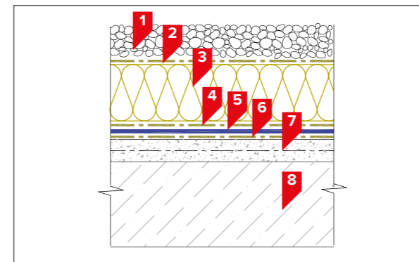
Рис. 2.8.4 Пример пирога инверсионной кровли
