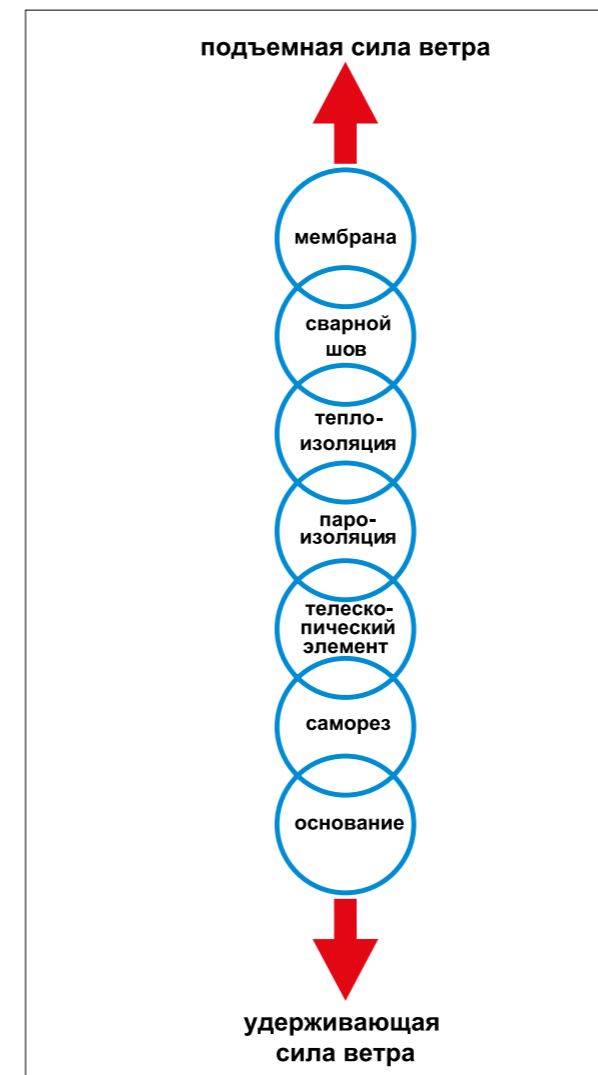
Рис. 3.5.3 Сопротивление подъемной силе ветра
