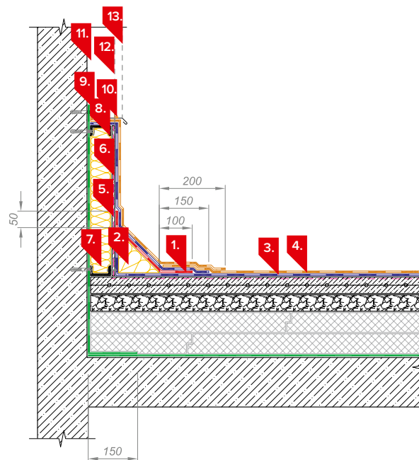
Рис. 7.7. Заведение пароизоляционного слоя к утепленным вертикальным конструкциям
