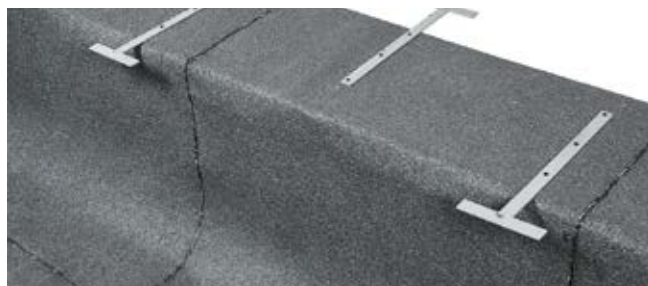
Рис. 7.28. Установка кровельных костылей
