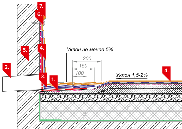
Рис. 7.55. Примыкание к парапетной воронки
