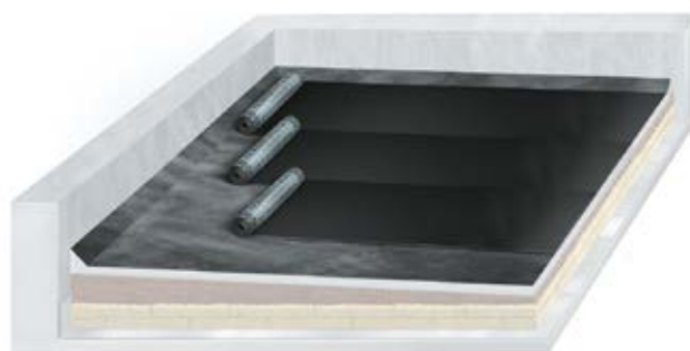
Рис. 7.17. 1 — Укладка материала перпендикулярно уклону при уклоне основания менее 15%;
