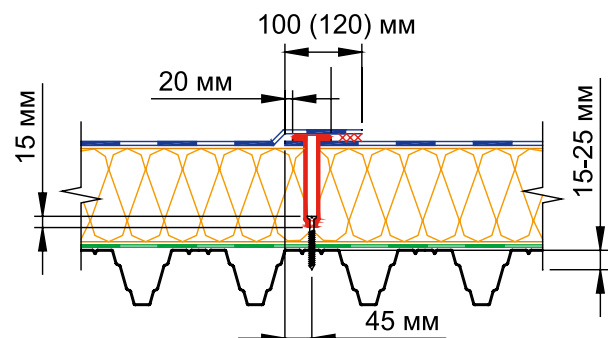
Рис. 7.43. Механическая фиксация материала в боковом нахлесте
