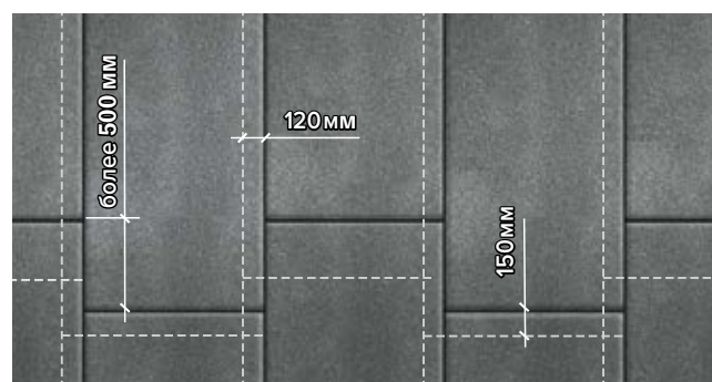
Рис. 7.50. Традиционное решение с разбежкой торцевых швов
