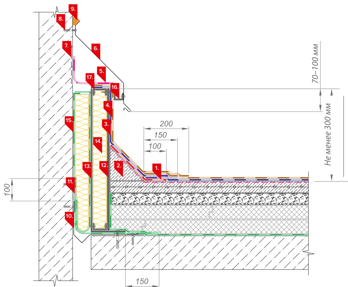
Рис. 7.60. Тип Д. Деформационный шов в месте сопряжения двух разновысоких частей здания:
