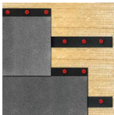
Рис. 7.45. Крепление полосы при устройстве однослойной кровли
