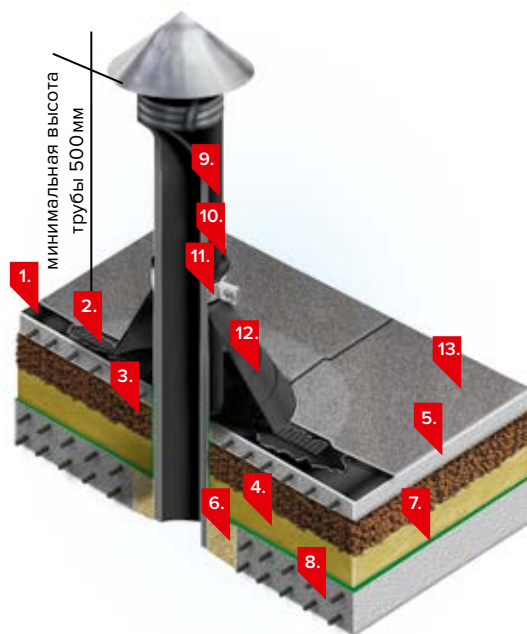
Рис. 7.31. Примыкание кровли к трубе с помощью эластичного переходника:
