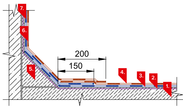
Рис. 7.18. Варианты раскладки водоизоляционного материала на переходном бортике при двухслойном водоизоляционном ковре.
