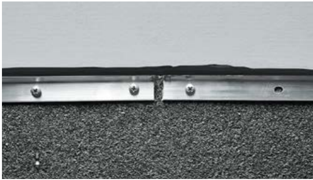
Рис. 7.21. Зазор между крайвыми рейками
