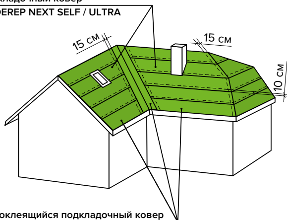
Самоклеящийся подкладочный ковер ANDEREP NEXT SELF / ULTRA
