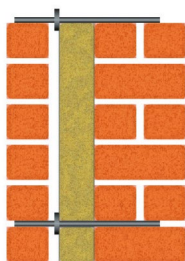
5. Ставятся базальто-пластиковые связи
