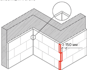
Рис. 29. Приклейка плиты тепло-, звукоизоляции к стене
