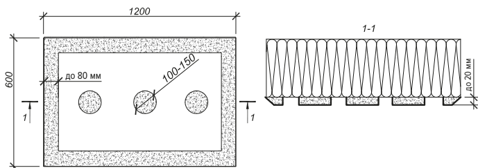
Рис. 28. Нанесение клея контурно-маячковым способом
