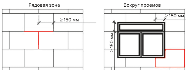
Рис. 31. Схема установки плит на плоскости фасада и вокруг проемов
