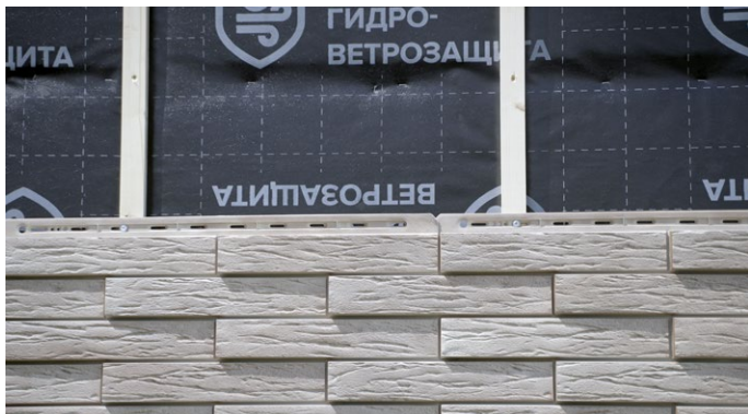
Рис. 22. Монтаж облицовочного материала
