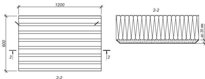
Рис. 27. Схема нанесения клея сплошным методом
