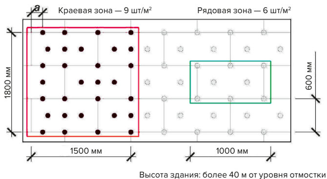
Рис. 33. Рекомендуемая схема расположения тарельчатых дюбелей на плоскости фасада в зависимости от высоты здания
