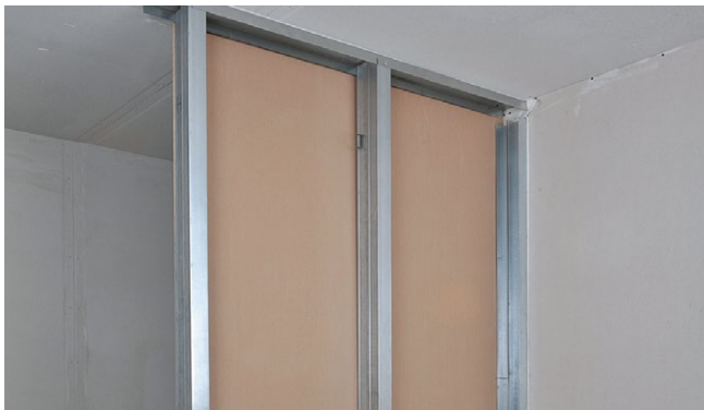
Рис. 5. Обшивка первой стороны перегородки листами ГКЛ
