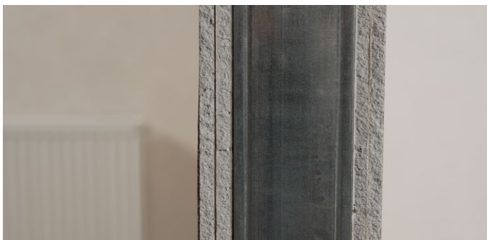
Рис. 7. Обшивка второй стороны перегородки листами ГКЛ
