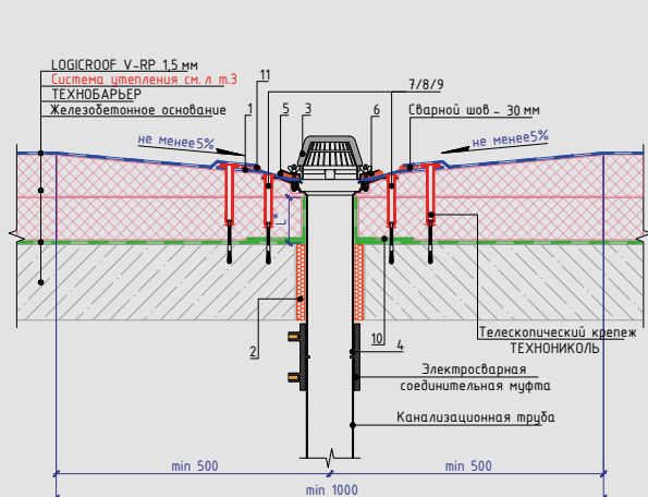
Устройство водоприемной воронки
