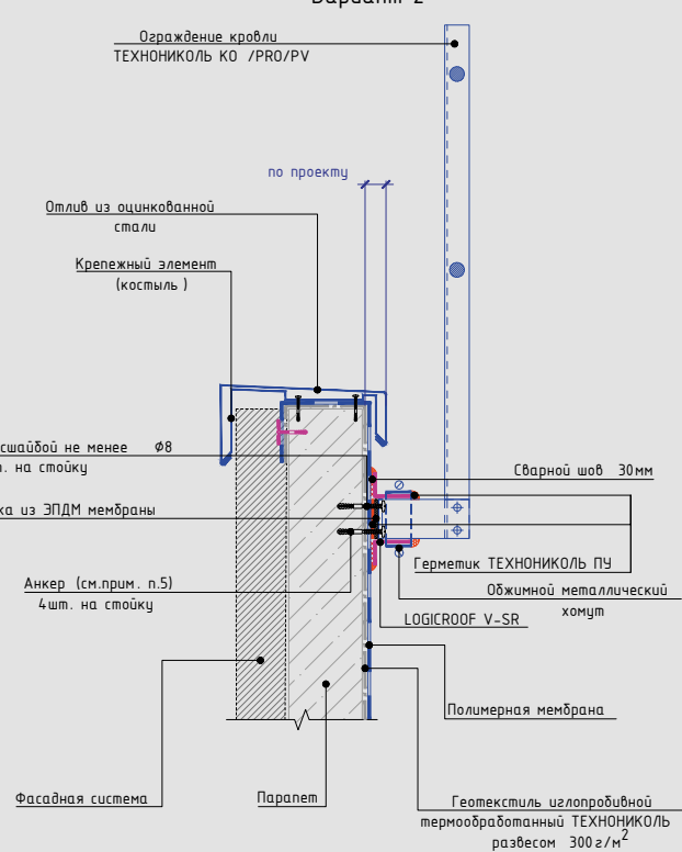
Схема крепления ограждения кровли ТЕХНИКОЛЬ КО/ПРО/РВ к бетонному парапету. Вариант 2
