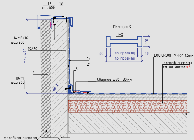
Примыкание к вертикальной поверхности с заведением ПМ за парапет
