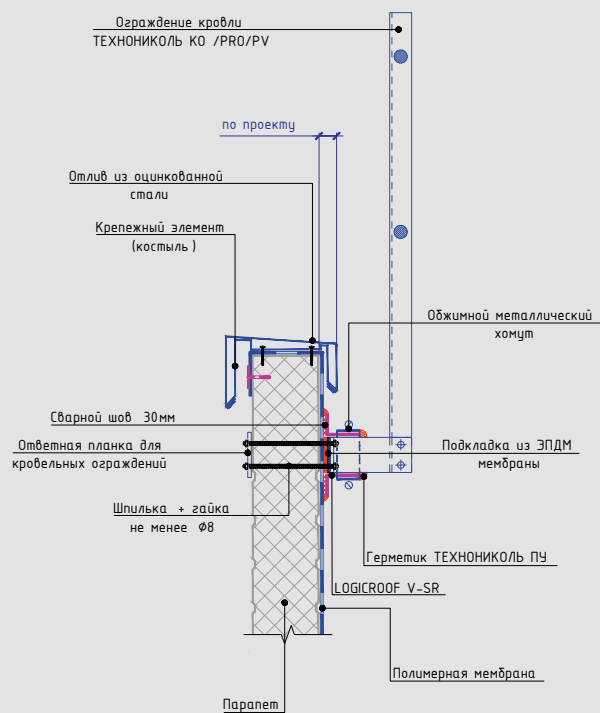
Схема крепления ограждения кровли ТЕХНИКОЛЬ КО/PRO/PV к парапету из сэндвич-панели
