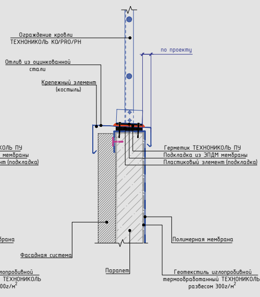
Схема крепления ограждения кровли к бетонному или каменному парапету. Вариант 3
