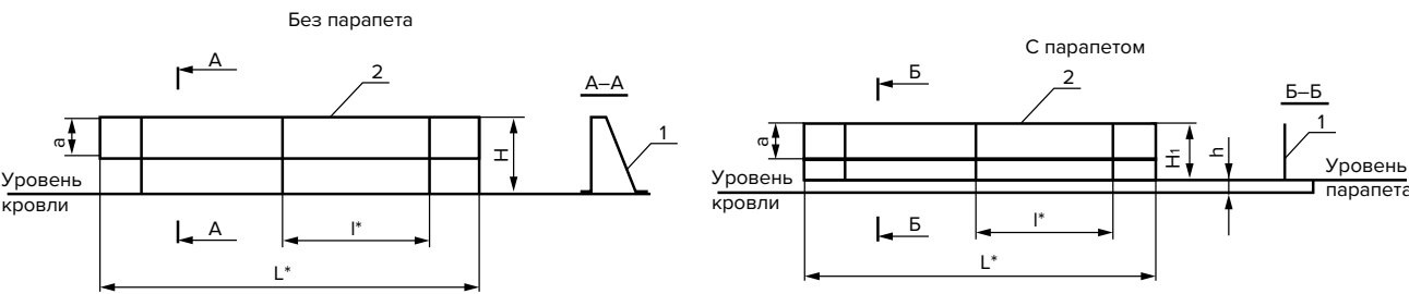
Рисунок Г.1 — Ограждения кровли 1 – вертикальный ограждающий элемент; 2 – горизонтальный ограждающий элемент * Настоящим стандартом не регламентируется.
