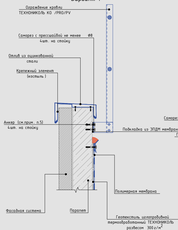
Схема крепления ограждения кровли ТЕХНИКОЛЬ КО/ПРО/РВ к бетонному парапету. Вариант 1
