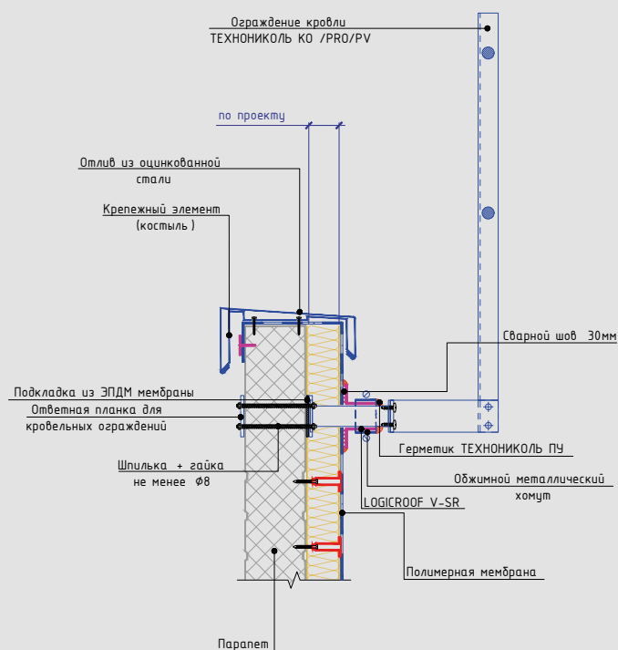
Схема крепления ограждения кровли ТЕХНИКОЛЬ КО/PRO/PV к парапету из сэндвич-панели
