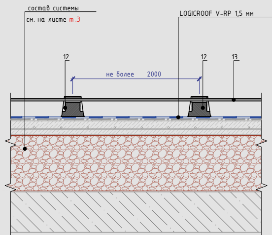
Устройство молниезащиты
