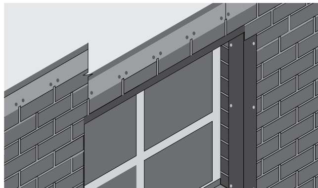
Рис. 15. Монтаж фасадной плитки поверх оконного наличника сверху проема
