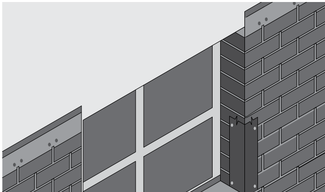
Рис. 12. Монтаж оконного наличника сбоку проема
