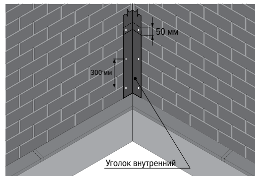
Рис. 24. Устройство внутренних углов
