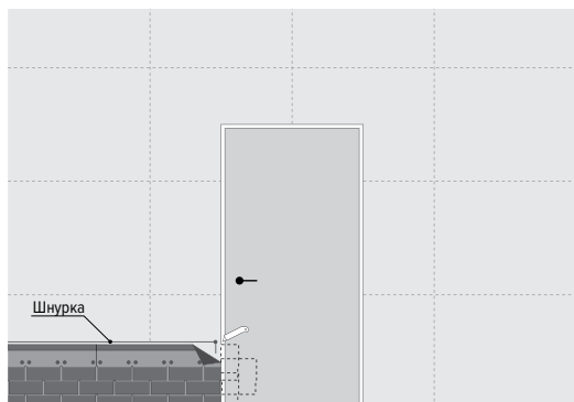
Рис. 8. Монтаж фасадной плитки вокруг дверных проемов
