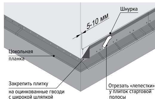
Рис. 6. Монтаж стартовой полосы фасадной плитки
