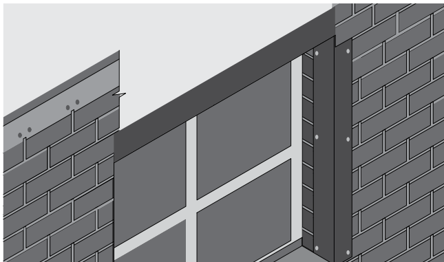
Рис. 14. Монтаж оконного наличника сверху проема
