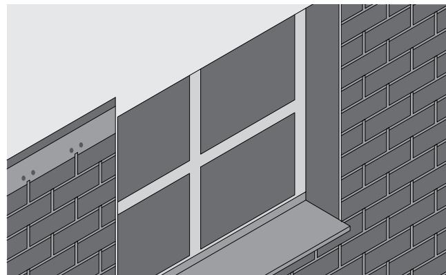
Рис. 11. Установка подоконного отлива
