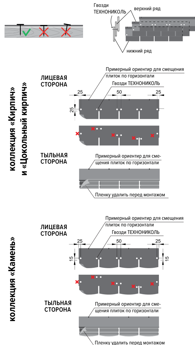
Рис. 2.1. Схема крепления фасадной плитки на 8 гвоздей
