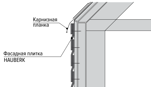
Рис. 27. Монтаж верхнего ряда в домах без карнизного свеса
