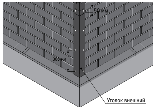
Рис. 23. Устройство внешних углов
