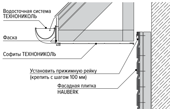
Рис. 25. Монтаж верхнего ряда под карнизным свесом. Вариант 1
