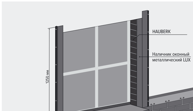
Рис. 17. Монтаж фасадной плитки вокруг оконных проемов
