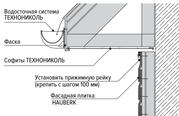
Рис. 26. Монтаж верхнего ряда под карнизным свесом. Вариант 2
