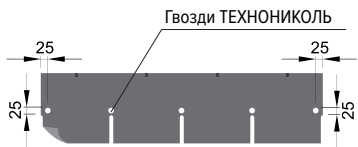
Рис. 3. Схема крепления фасадной плитки на 5 гвоздей
