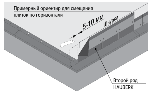
Рис. 7. Монтаж первого и последующих рядов фасадной плитки
