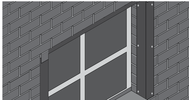
Рис. 16. Законченный вид
