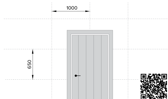
Рис. 5. Разметочные линии
