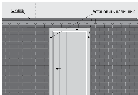
Рис. 9. Установка наличников
