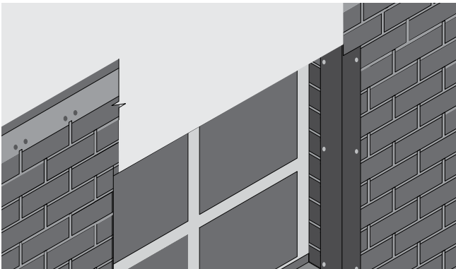
Рис. 13. Монтаж бокового наличника (верхний край заходит под фасадную плитку)
