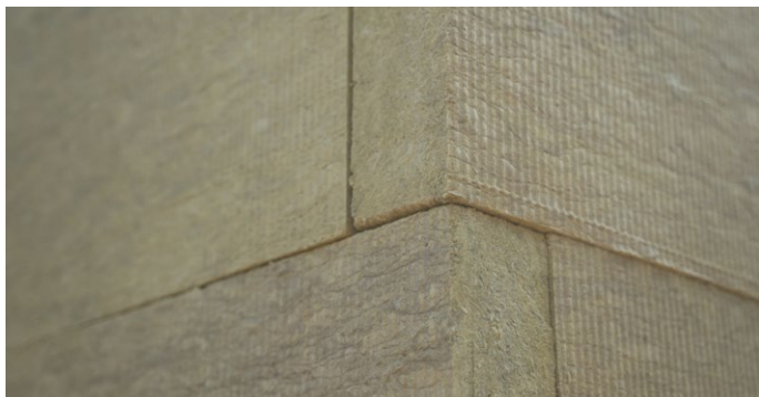
Рис. 10. Зубчатая перевязка плит на наружных углах здания
