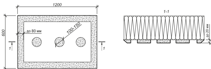
Рис. 7. Схема точечного (контурно-маячкового) нанесения клея на плиту
