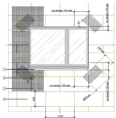
Рис. 14. Схема установки усиливающих элементов из армирующей сетки вокруг дверных и оконных проемов
