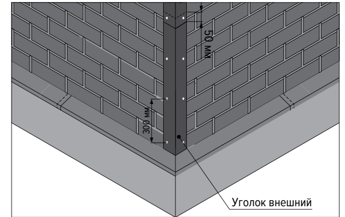
Рис. 9. Устройство внешних углов
