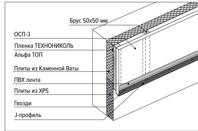
Рис. 6. Монтаж J-профиля
