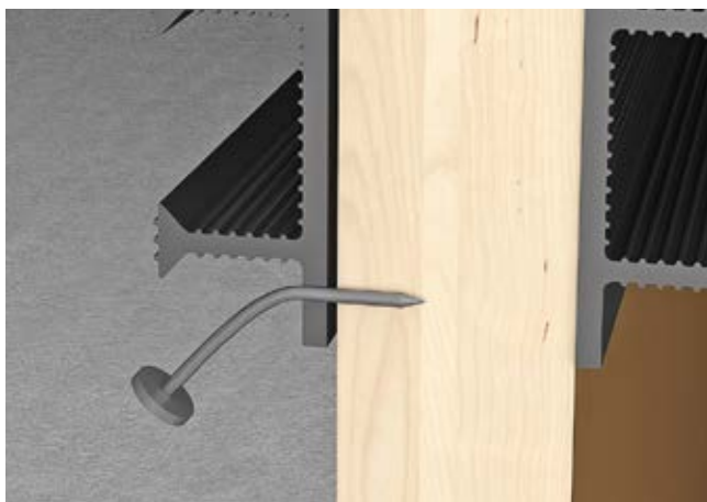
Рис. 4.4. Крепление боковых и П-образных гидрошпонок к опалубке с помощью гвоздей
