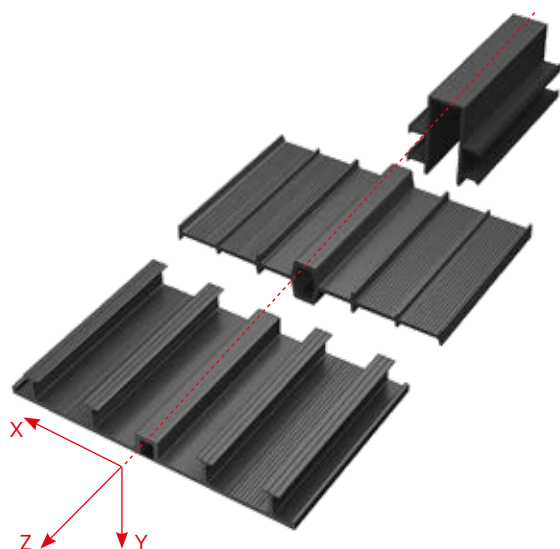
Рис. 3.4. Деформации гидрошпонок в различных плоскостях
