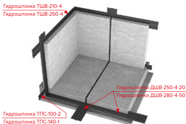
Рис. 3.2а. Замкнутый гидроизоляционный контур с применением внутренних гидрошпонок
