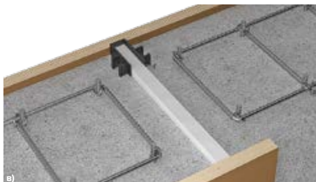
Рис. 5.4. Этапы работ по установке гидрошпонок серии ТН Фундамент ДШП
