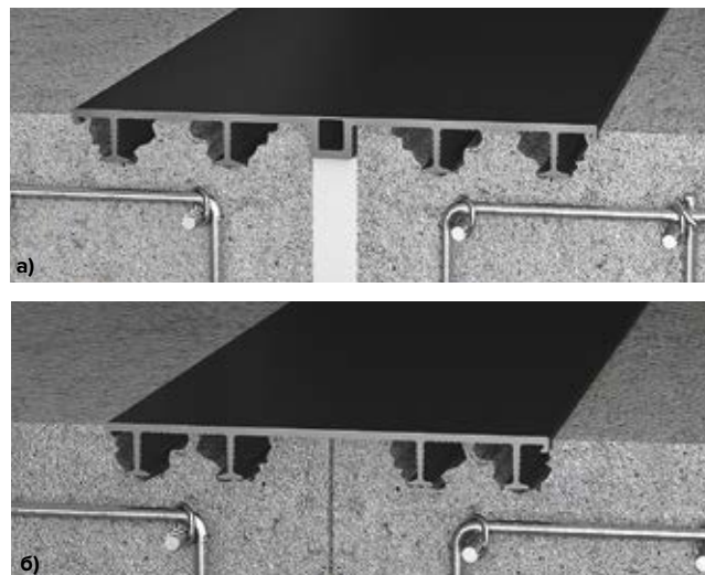
Рис. 3.9. Дефекты омоноличивания, возникающие при установке наружных гидрошпонок в верхнюю часть горизонтальных конструкций
