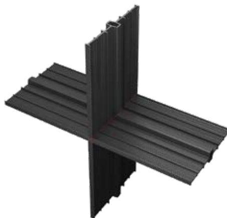
Рис. 4.12. Фасонный элемент: вертикальный крестообразный стык (рекомендуется выполнять на оборудованном посту)
