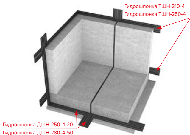
Рис. 3.2б. Замкнутый гидроизоляционный контур с применением наружных гидрошпонок
