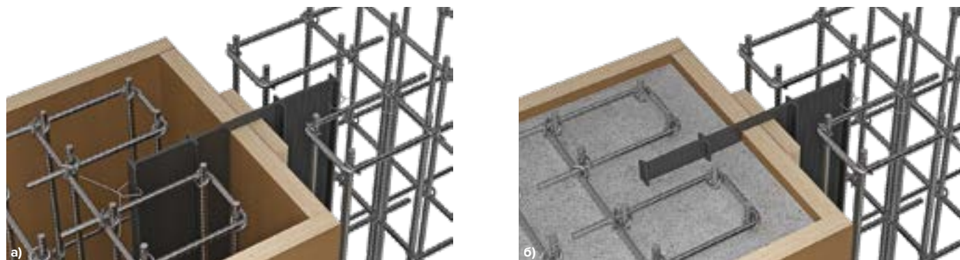
Рис. 5.3а,б. Этапы работ по установке гидрошпонок серии ТН Фундамент ТШВ
