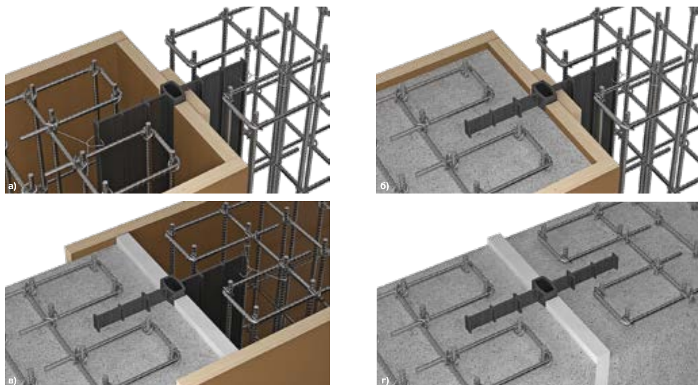
Рис. 5.2. Этапы работ по установке гидрошпонок серии ТН Фундамент ДШВ
