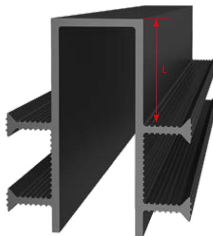
Рис. 3.5. П-образная гидрошпонка
