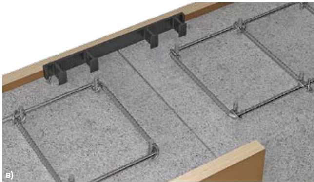
Рис. 5.6. Этапы работ по установке гидрошпонок серии ТН Фундамент ТШН
