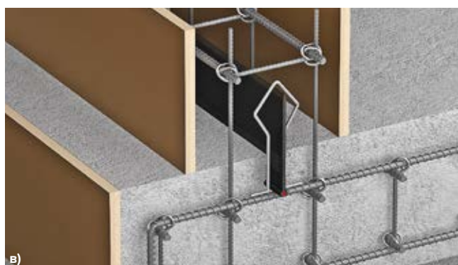
Рис. 5.3. Этапы работ по установке гидрошпонок серии ТН Фундамент ТПС
