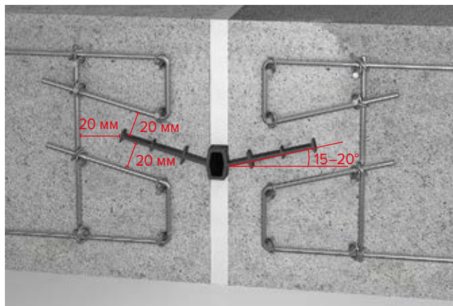
Рис. 3.11. Установка внутренних гидрошпонок под углом
