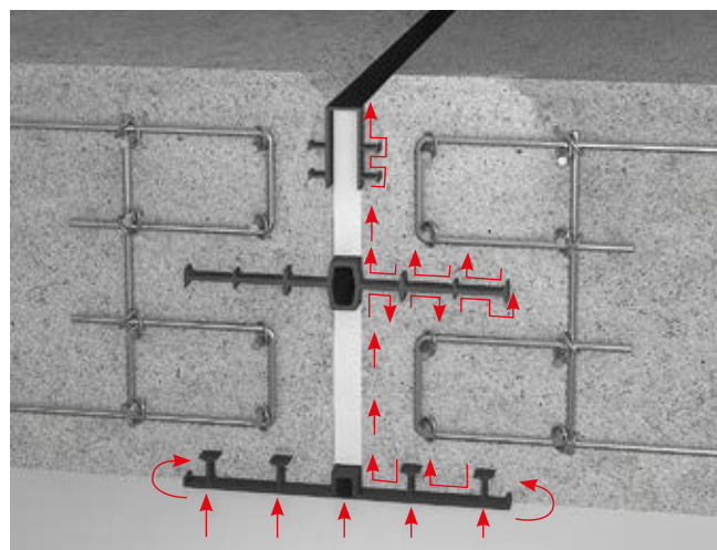
Рис. 3.1. Принцип работы гидрошпонки
