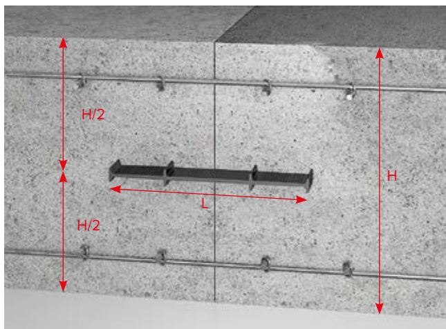
Рис. 3.6. Подбор ширины гидрошпонки, правило Перекрытия
