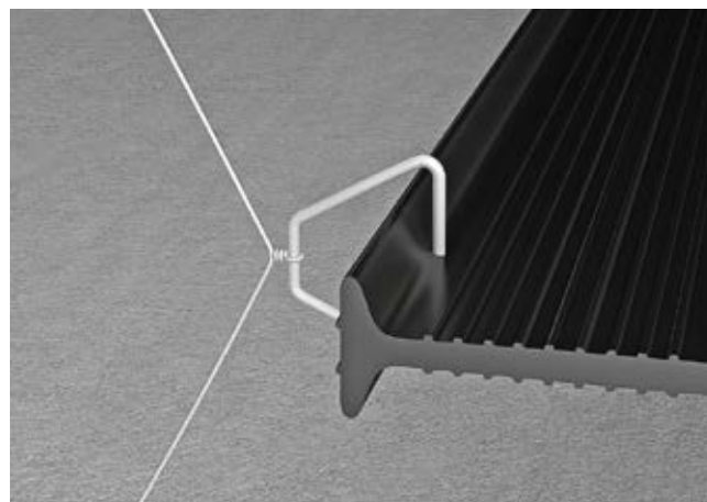
Рис. 4.3. Установка внутренних гидрошпонок с помощью специальных крепежных клипс
