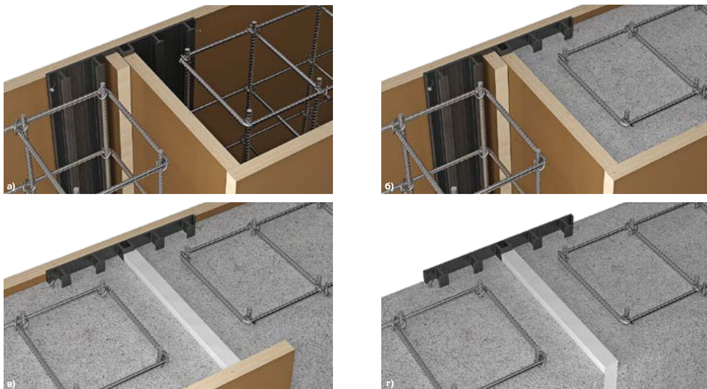
Рис. 5.5. Этапы работ по установке гидрошпонок серии ТН Фундамент ДШН
