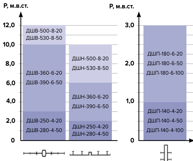
Рис. 3.7. Подбор профиля и размера гидрошпонок исходя из давления воды на узел деформационного шва
