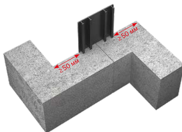
Рис. 3.14. Расстояние от края наружных гидрошпонок до угла конструкций
