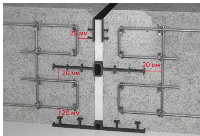
Рис. 3.10. Расстояние от края гидрошпонки до арматурного каркаса
