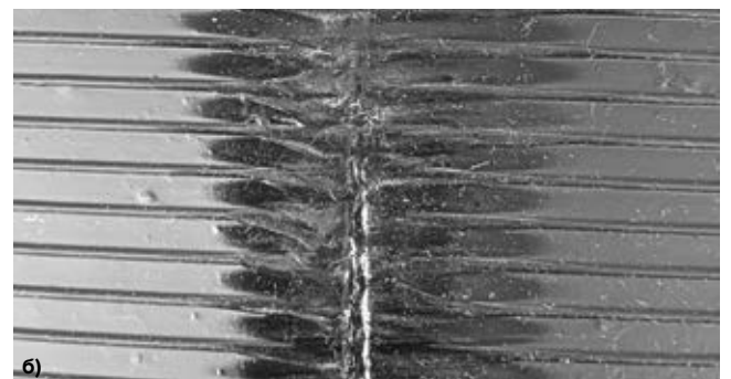
Рис. 4.15. Сварные соединения гидрошпонок а) с валиком вытека (при применении сварочного утюга и топорика) б) без валика вытека (при применении электрического фена)
