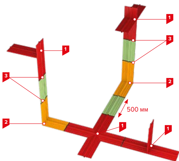
Рис. 3.12. Категории монтажных стыков гидрошпонок
