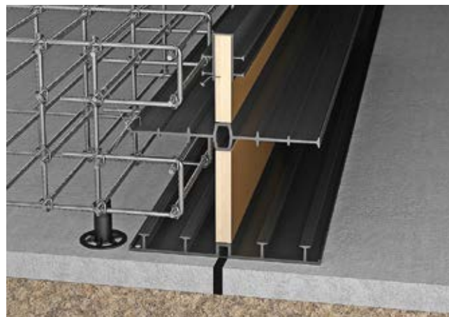
Рис. 4.2. Установка различных типов гидрошпонок в проектное положение
