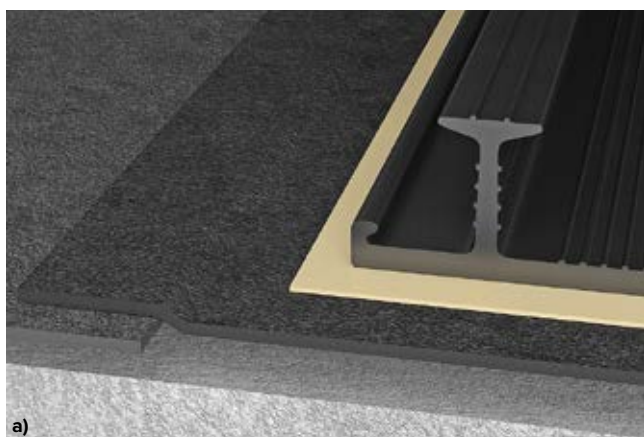
Рис. 4.5. Варианты установки наружных гидрошпонок на горизонтальную поверхность а) на клеевой состав /ленту б) методом механической фиксации
