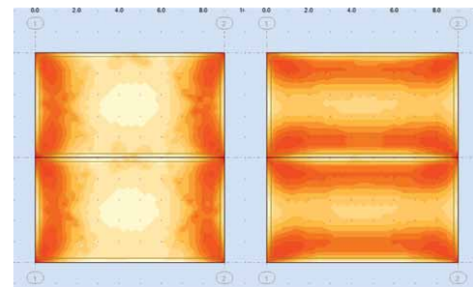
Рисунок 7.4 Карты армирования УШП в верхней зоне
