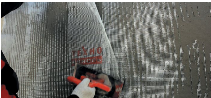
Рис. 37. Армирование базового штукатурного слоя стеклосеткой
