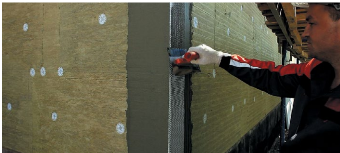
Рис. 35. Установка усиливающих профилей на углах здания
