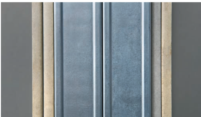
Рис. 7. Обшивка второй стороны перегородки листами ГКЛ
