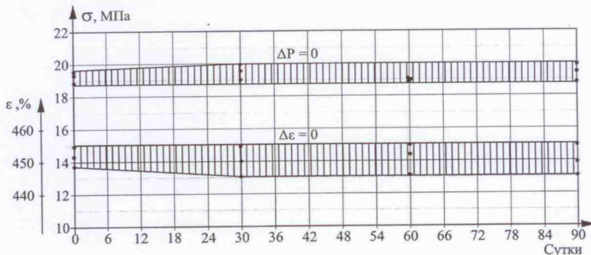
Рис. 1. Изменение прочности (1) и относительного удлинения (2) образцов рулонного материала "LOGICROOF T SL 1,5 мм" при воздействии 15-% раствора NaOH
