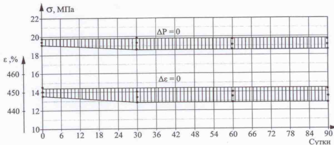
Рис. 2. Изменение прочности (1) и относительного удлинения (2) образцов рулонного материала "LOGICROOF T SL 1,5 мм" при воздействии 15-% раствора H_2SO_4
