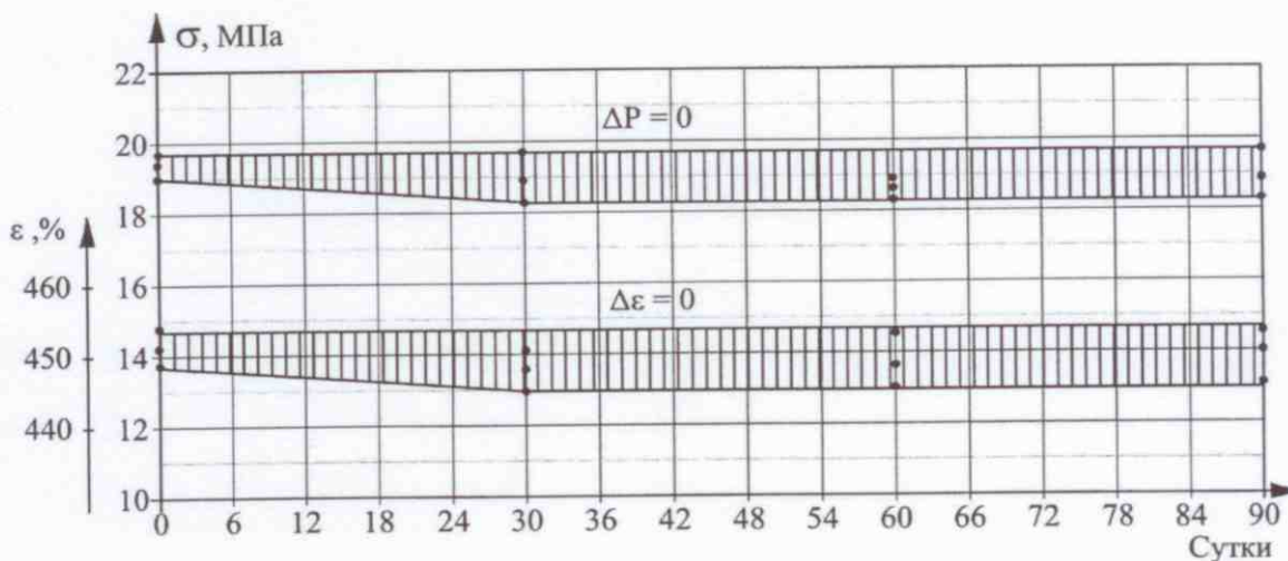
Рис. 3. Изменение прочности (1) и относительного удлинения (2) образцов материала "LOGICROOF T SL 1,5 мм" при воздействии насыщенного раствора NaCl
