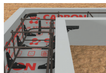
Ленточный фундамент
