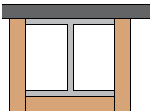
Трехсторонняя изоляция \Pi = 2H + S (m)
