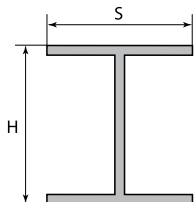
Двутавровый профиль S — ширина подошвы профиля H — общая высота профиля
