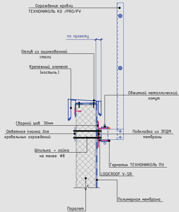
Схема крепления ограждения кровли ТЕХНИКОЛЬ КО/ПРО/ПВ к парапету из сэндвич-панели
