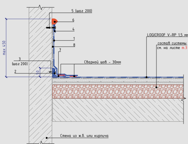
Примыкание к вертикальной поверхности (вент. шахты, вент. блоки, тамбуры выхода на кровлю, лифтовые шахты и прочее)
