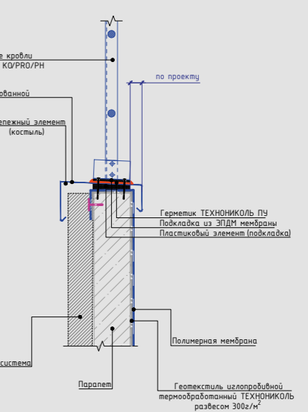
Схема крепления ограждения кровли к бетонному или каменному парапету. Вариант 3
