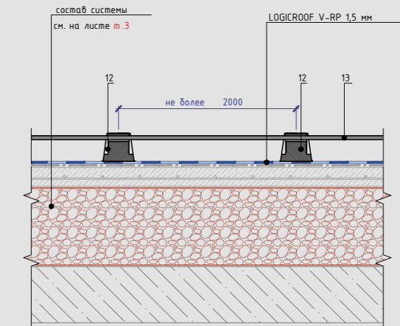
Устройство молниезащиты
