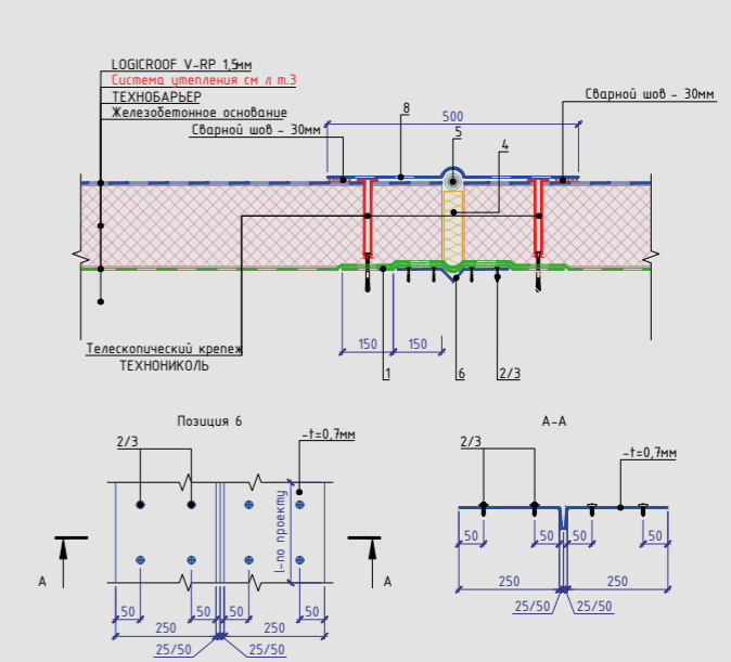
Устройство деформационного шва
