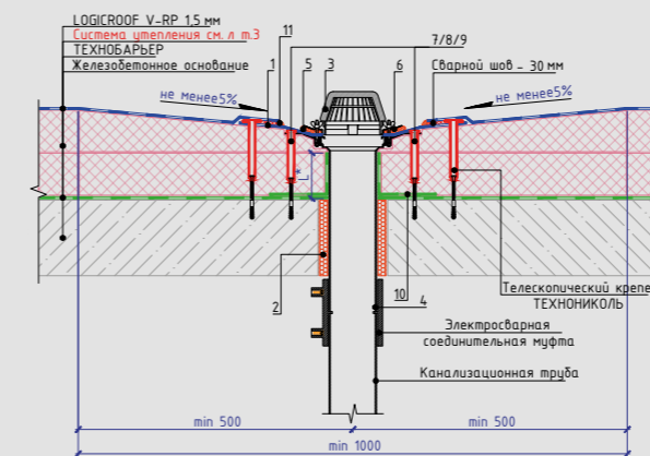
Устройство водоприемной воронки
