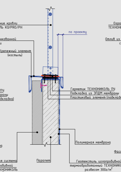
Схема крепления ограждения кровли к бетонному или каменному парапету. Вариант 2
