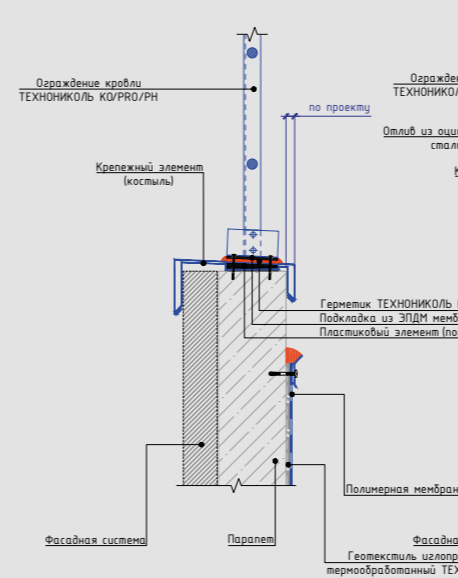
Схема крепления ограждения кровли к бетонному или каменному парапету. Вариант 1
