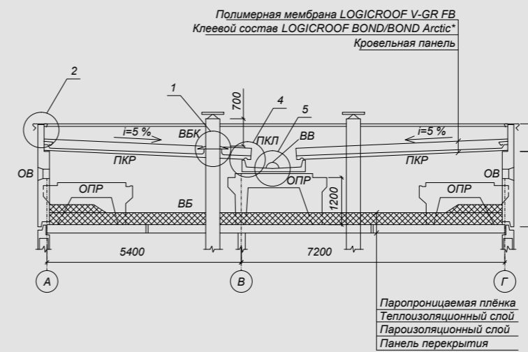
Устройство гидроизоляции лотковых кровель
