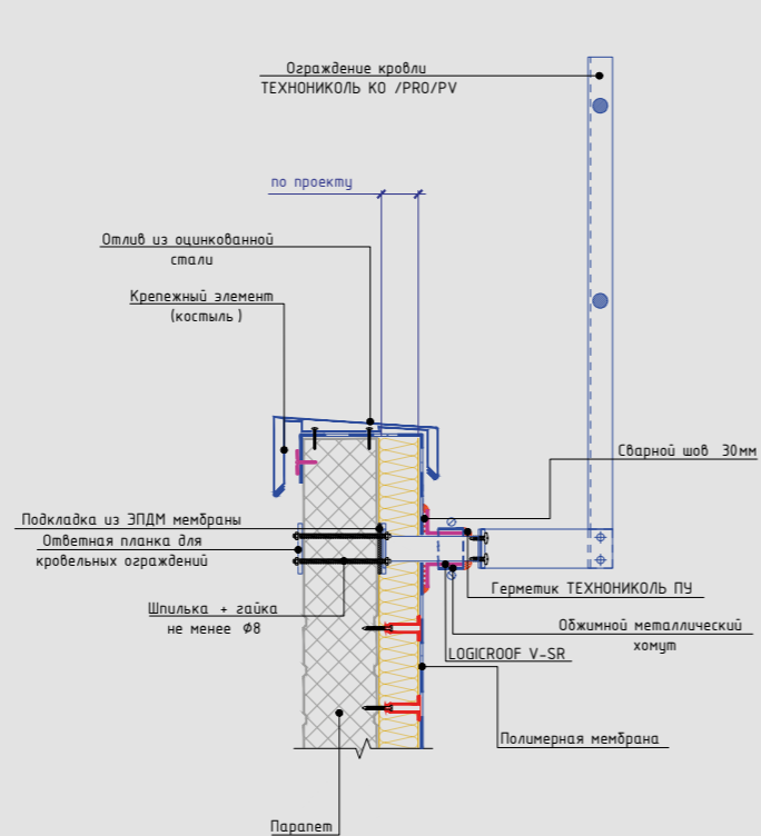
Схема крепления ограждения кровли ТЕХНИКОЛЬ КО/ПРО/ПВ к парапету из сэндвич-панели
