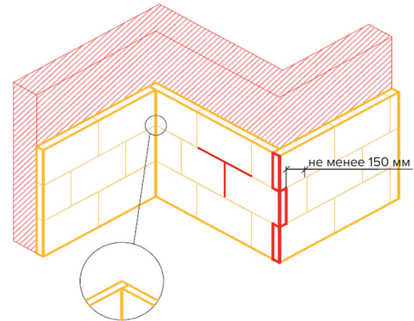
Расположение утеплителя в углах проемов
