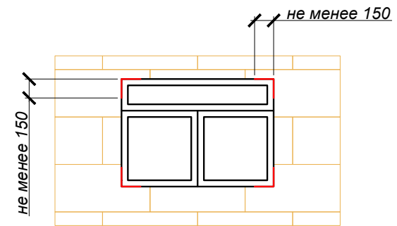
Расположение утеплителя в углах проемов
