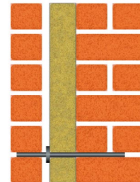
4. Укладывается теплоизоляция
