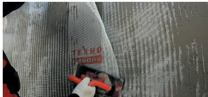
Рис. 37. Армирование базового штукатурного слоя стеклотеткой
