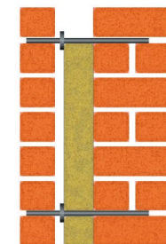
6. Кладется один ряд поверх связей в обоих слоях
