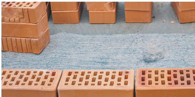
Рис. 7. Гидроизоляционная отсечка
